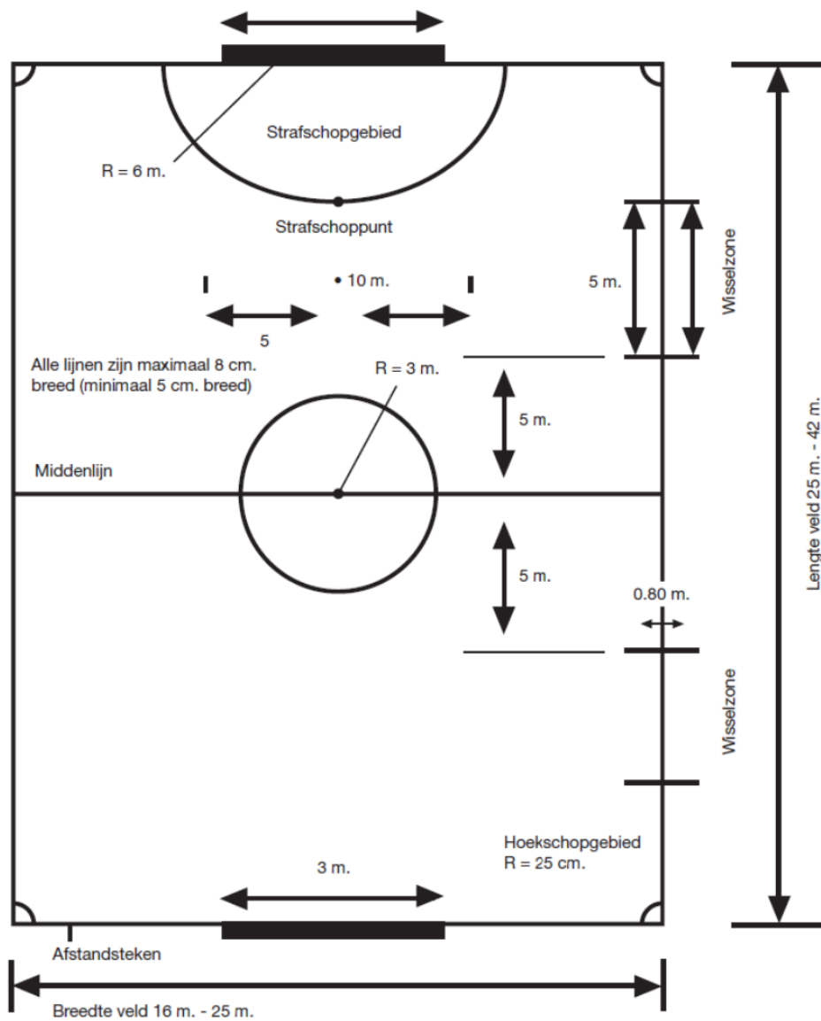
Figuur speelveld zoals opgenomen in Spelregels Top- en Eredivisie futsal juli 2011.
